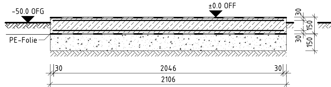
Schnitt A-B M 1:20
