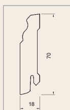
Querschnitt: Sockelleiste VWDE3110 / VWDE3112
