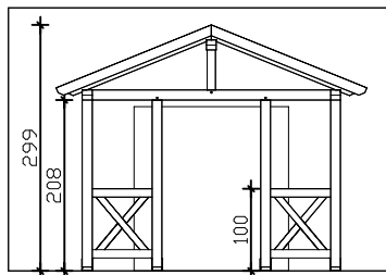
Frontansichten
