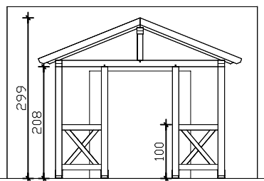
Frontansichten
