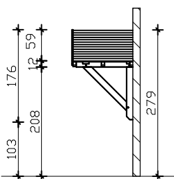
Seitenansichten
