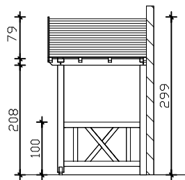
Seitenansichten
