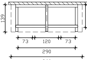
Grundrisse
