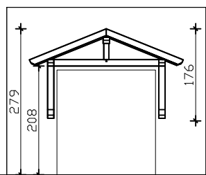
Frontansichten
