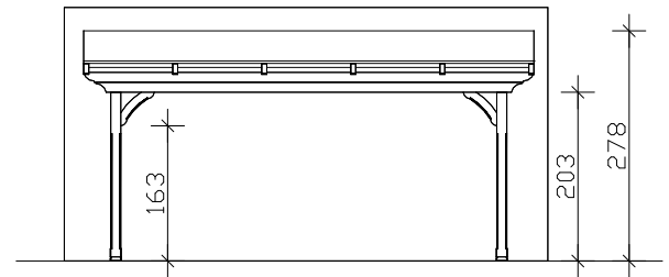
Frontansicht
