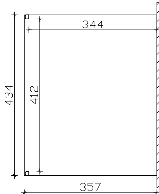
Grundriss
