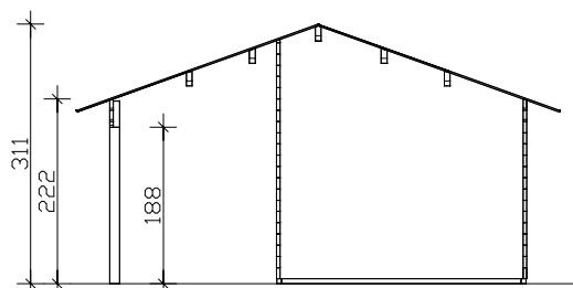
Grundriss, Schnitt und Ansichten M 1:100
