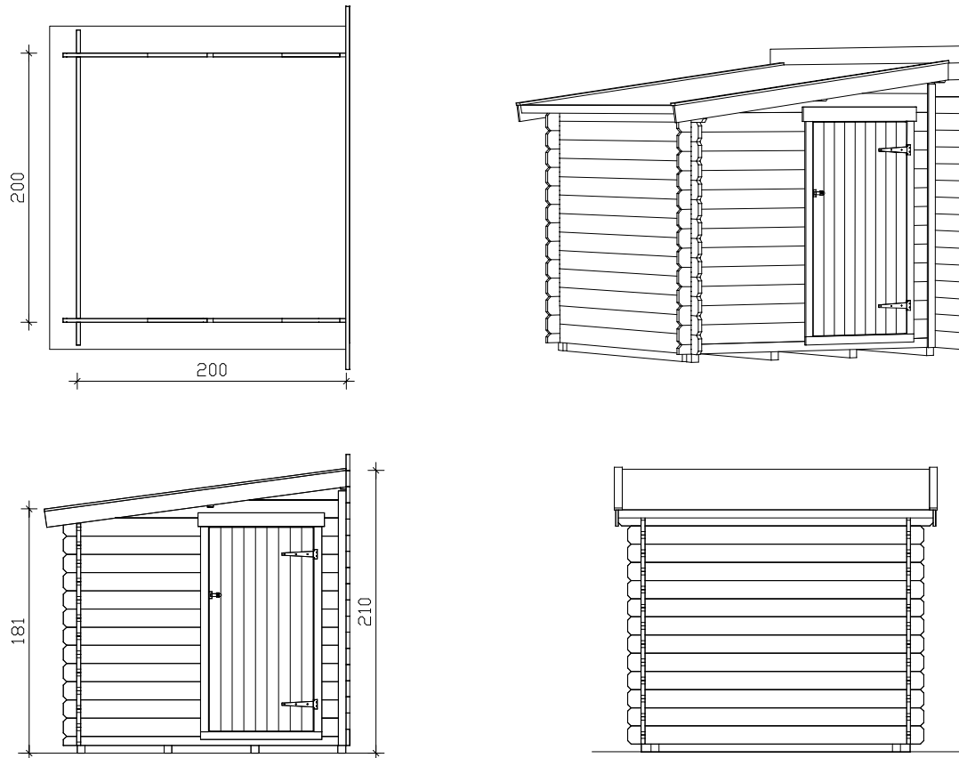
Grundriss, Schnitt und Ansicht M 1:50
