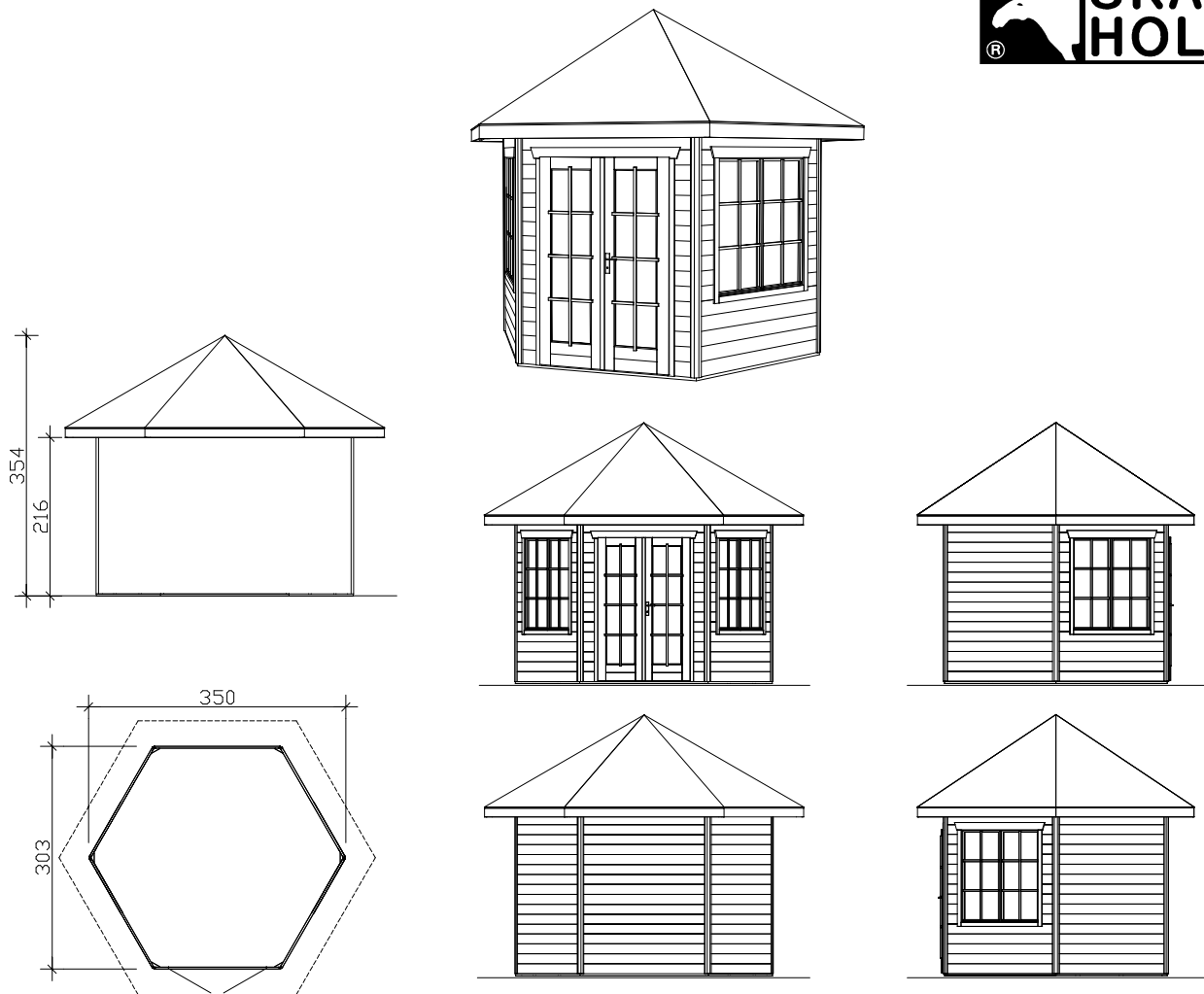
Grundriss, Schnitt und Ansichten M 1:100
