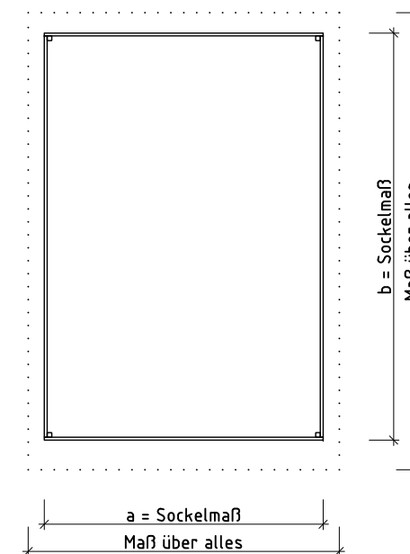
Grundriss M 1:50
