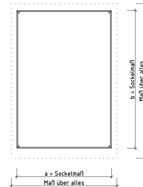
Grundriss M 1:50
