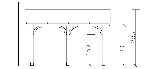
Fronansicht
