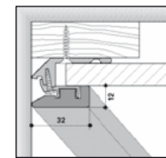
Abschlussleiste
