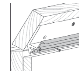
Halteleiste montieren
