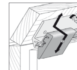
Befestigungsschiene positionieren
