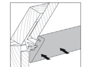
HDF-Leiste aufstecken
