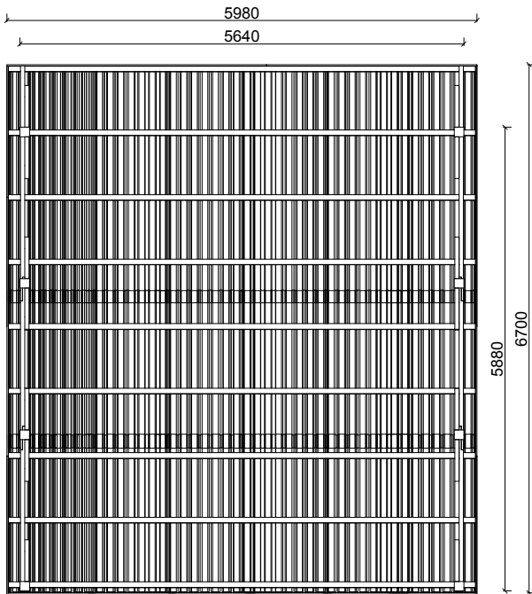
Grundriss
