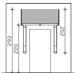
Frontansichten
