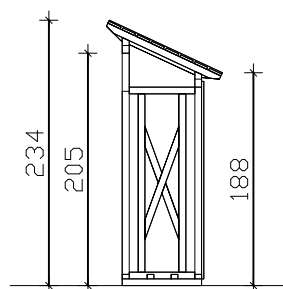
Schnitt
