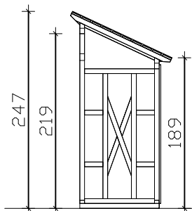
Schnitt
