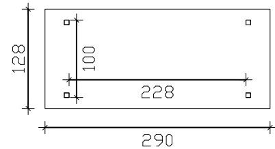
Grundriss
