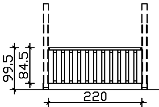
Bemassung
