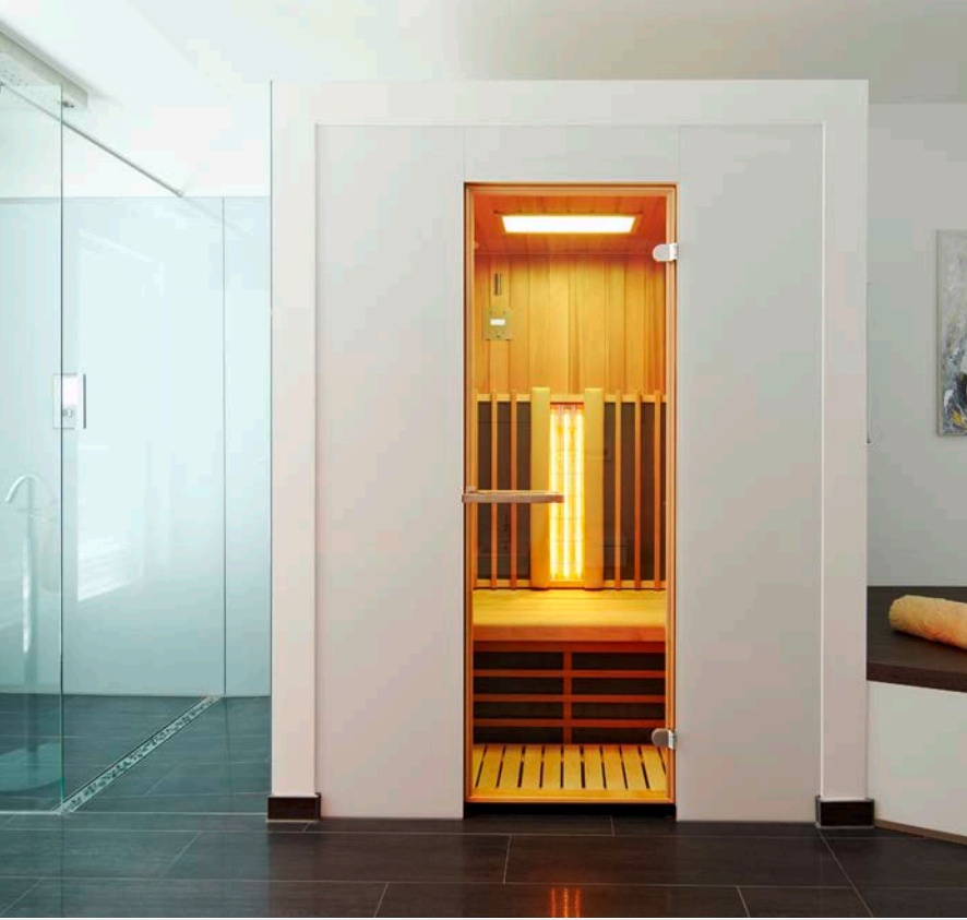
Abbildung TrioSol Infrarotkabine in Maßanfertigung: Sondermaß bei Breite und Tiefe, Holzart kanadische Zeder, VITAllight-Infrarotstrahler in der Kabinenmitte positioniert, Flächenheizung anthrazit. Die Verkleidung der Vorderfront mit weißen Glaspaneelen erfolgte durch den Fachhändler.
