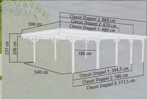
1 DOPPELCARPORT CLASSIC 2, KDI, mit Zubehör (gegen Aufpreis): 8 Pfostenanker
