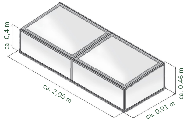
FRÜHBEET 210
