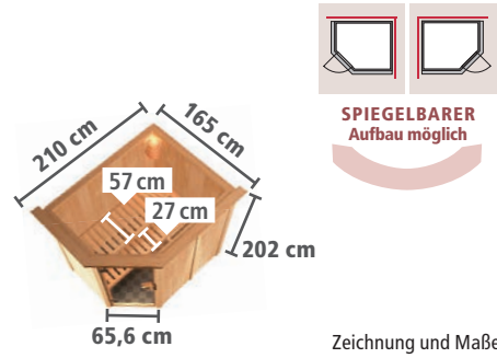
Abb. CARIN mit Dachkranz und Zubehör (gegen Aufpreis): Saunaleuchte Premium und Bodenrost
