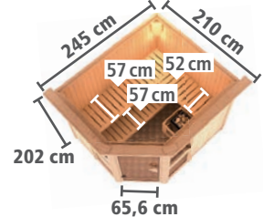
Zeichnung und Maße mit Dachkranz
