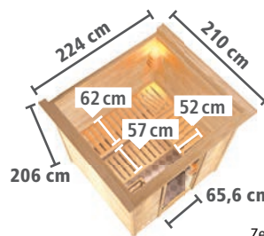
Abb. MOJAVE mit Dachkranz und Zubehör (gegen Aufpreis)
