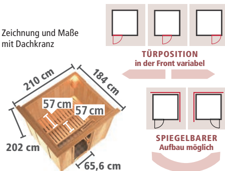
Abb. DARIA mit Dachkranz und Zubehör (gegen Aufpreis)
