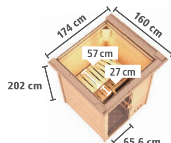
Zeichnung und Maße mit Dachkranz
