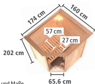
Zeichnung und Maße mit Dachkranz
