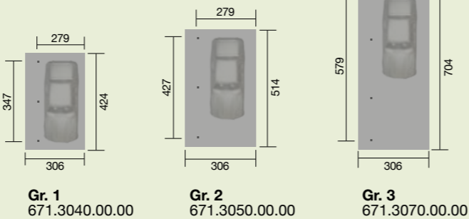
Anlehn-Carport 671 (je nach Größe unterschiedliche Pfostenanzahl, siehe Grundriss)
