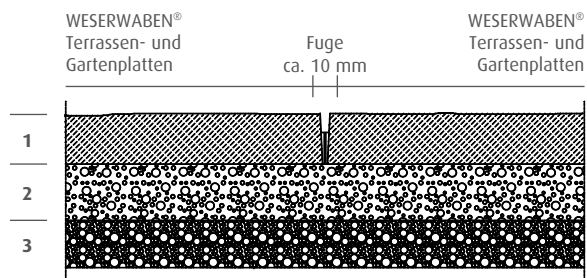
Abb. 2: Prinzip-Skizze Terrassenplatte Scivaro
