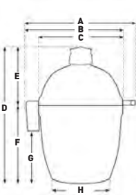
SEITENANSICHT
