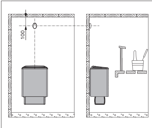
Figure 8. Installing the sensor (all dimensions in millimeters) Abbildung 8. Installation der Fühler (alle Abmessungen in Millimetern)
