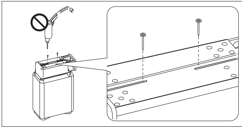
Figure 5. Removal of the end-piece fastening screws Abbildung 5. Lösen der Befestigungsschrauben der Stirnstücke
