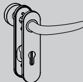
Kurzschild WG mit Knopf Ausführungen: Kl 4 / FS (Vierkant 9 mm) Schlüsselbohrungen: PZ, PZ FS
