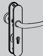
Langschild WG Panik mit Knopf R2 Ausführungen: FS (Vierkant 9 mm) Schlüsselbohrungen: PZ FS
