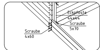
2 Schrauben für Bohle
