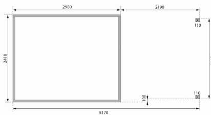
Fundamentplan ohne Boden (in mm)
